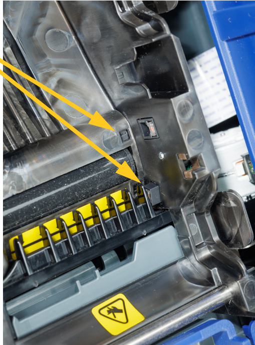
Abbildung 2-2. Position der Vorderkante des Etikettenverbrauchsmaterials.
